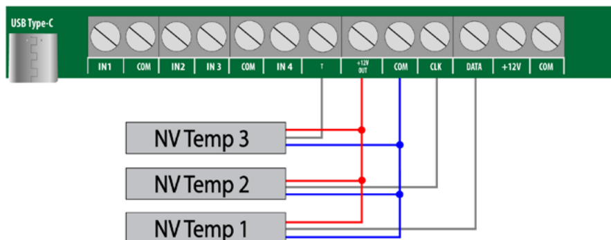
Рисунок 2. Подключение датчиков температуры NV TEMP
