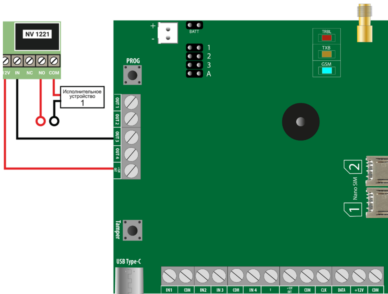
Рисунок 5. Пример подключения NV 1221 к выходу NV 8316
