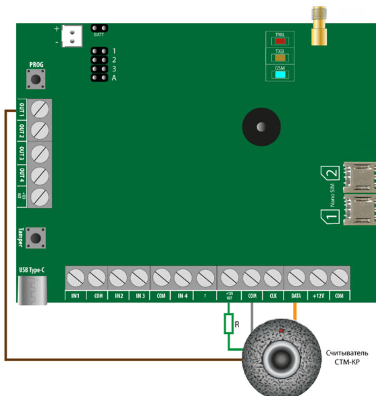
Рисунок 3. Схема подключения на примере ТМ считывателя CTM-KT
