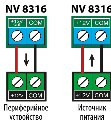
Рисунок 1. Подключение питания
